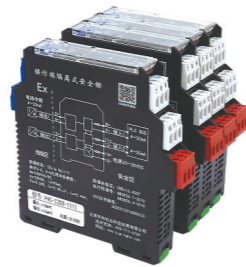
D 系列 液晶显示型 隔离式安全栅 D SERIE OLED ISOLATED SAFETY BARRIERS
